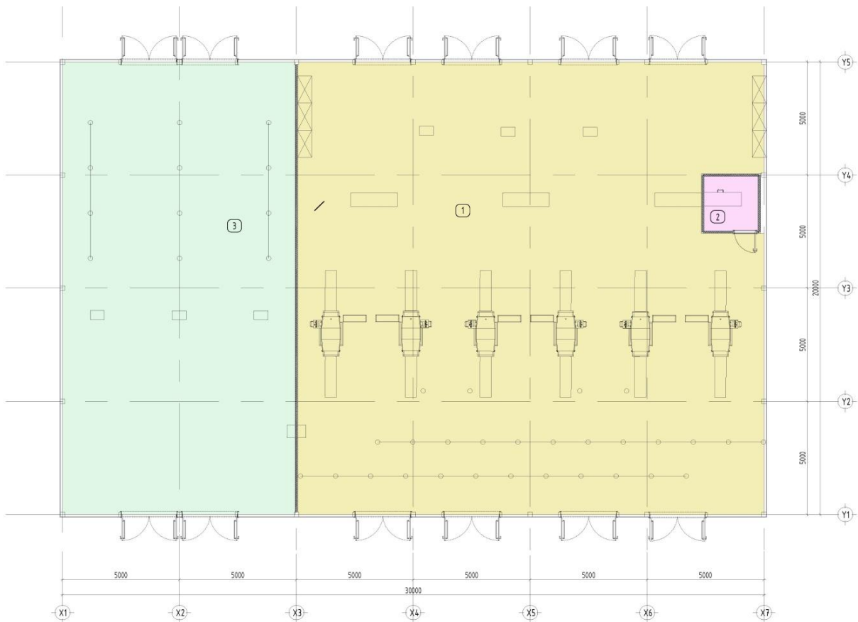
/Зураг 3. Холбох байгууламжийн ерөнхий төлөвлөлт/
