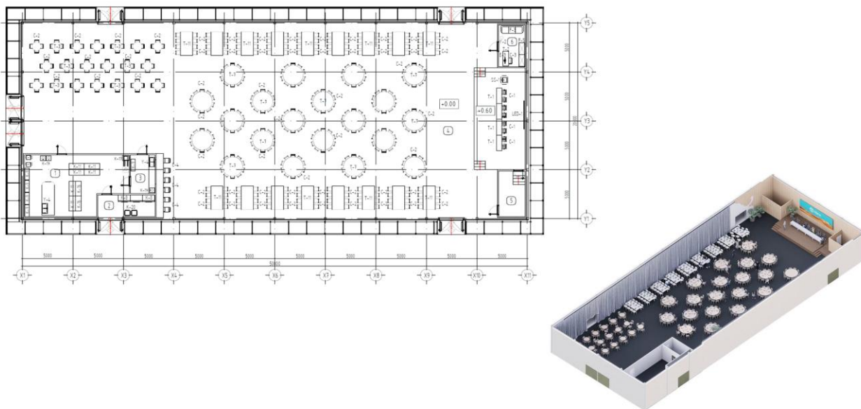
/Зураг 2. Хүлээн авалтын танхимын ерөнхий төлөвлөлт/
